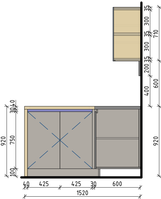
Боковой вид
