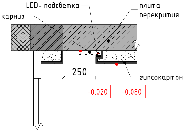
Разрез 3-3
