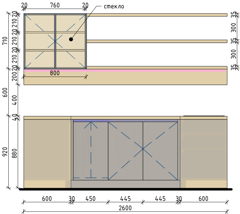
Фронтальный вид
