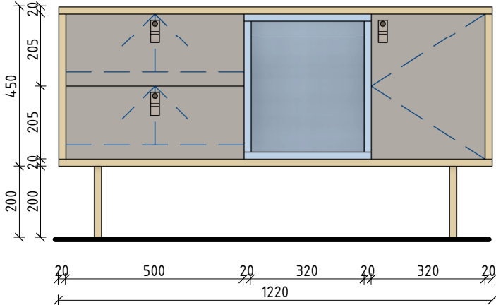
Фронтальный вид
