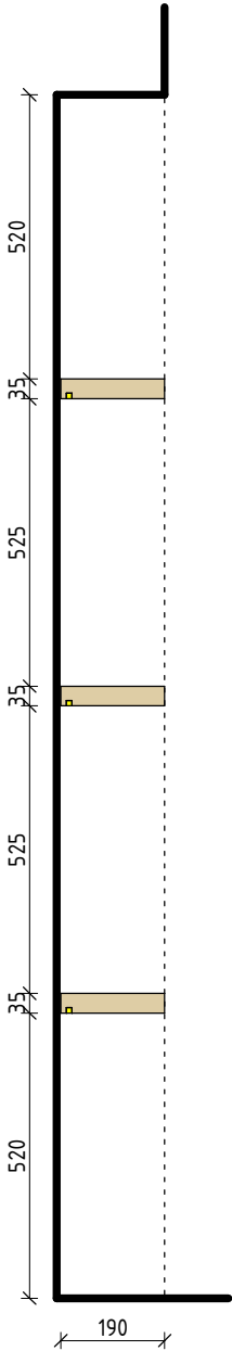
Боковой вид
