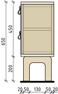
Боковой вид
