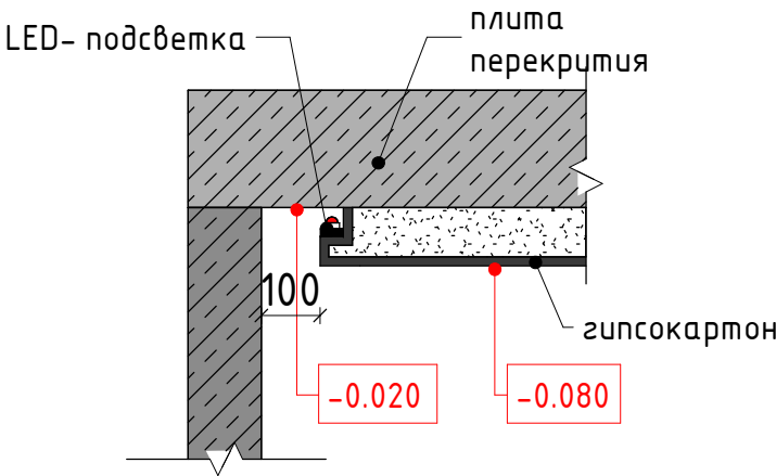
Разрез 1-1
