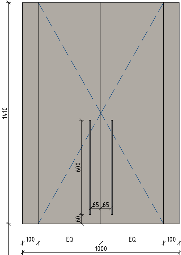
Фронтальный вид
