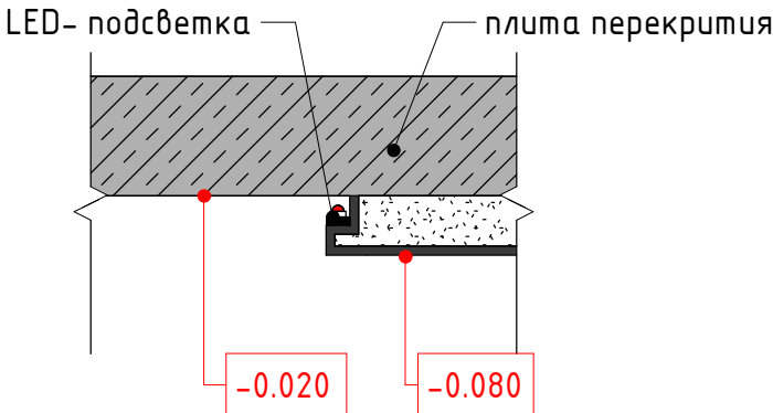
Разрез 4-4
