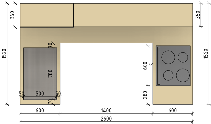
Вид сверху
