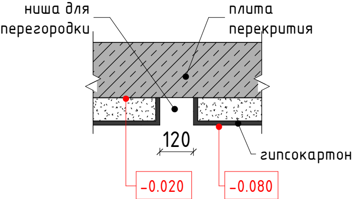
Разрез 2-2
